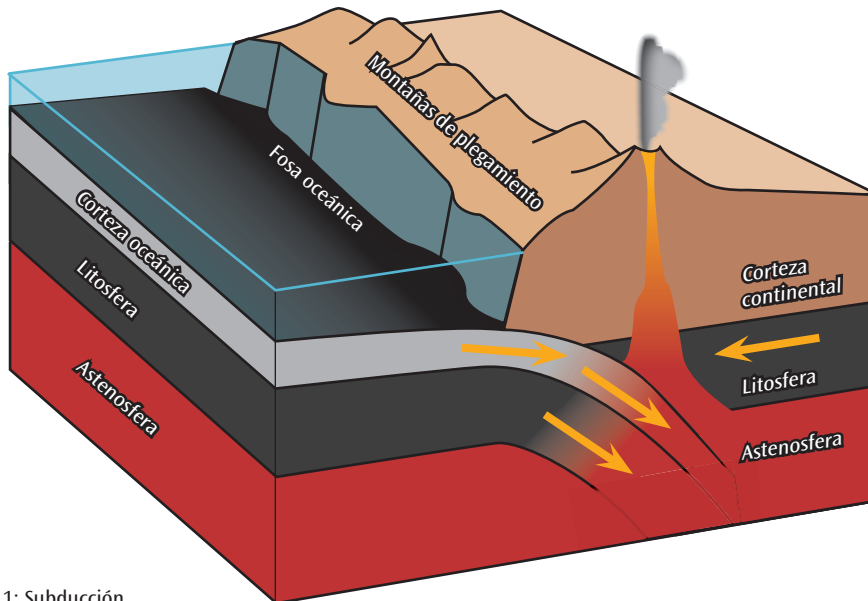
Ilustración 1: Subducción
