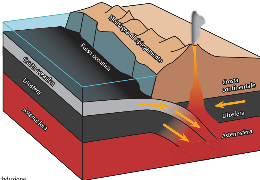
Figura 1: subduzione
