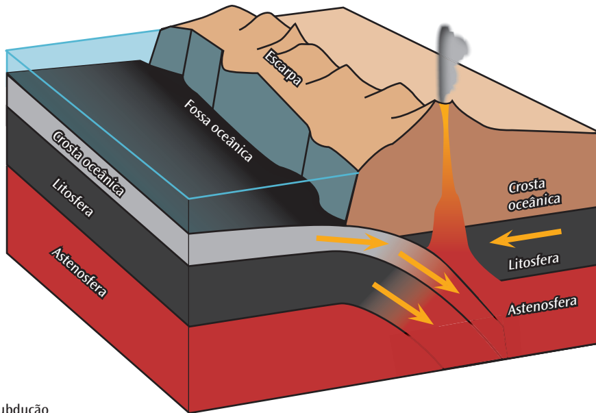
Figura 1: Subdução
